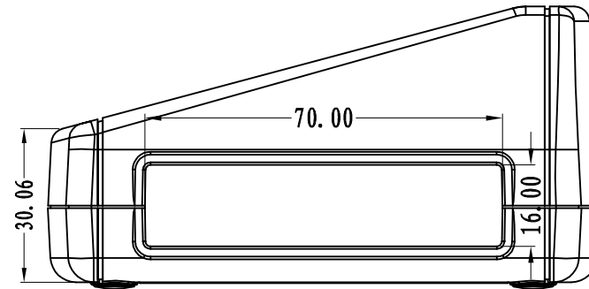
SEC A-A
