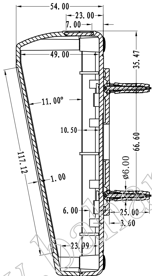
SEC A-A
