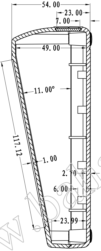
SEC A-A
