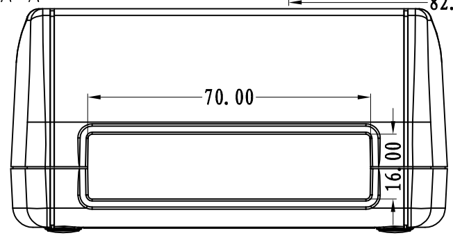
SEC A-A
